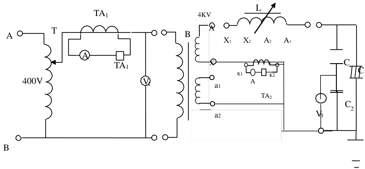
图 7 串联谐振试验原理接线图
