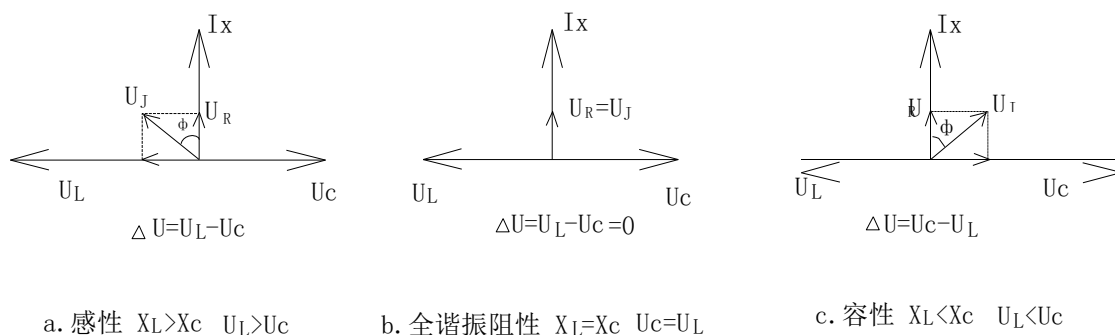
图 2 R、L、C 串联电路向量图
