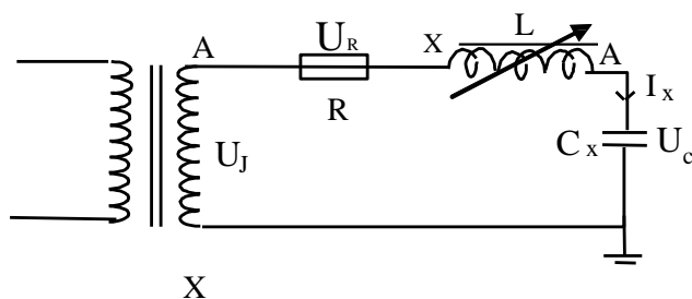
图 1 串联谐振回路原理图 L——可调电抗器的电感量 C x ——被试品电容量 R——可调电抗器
