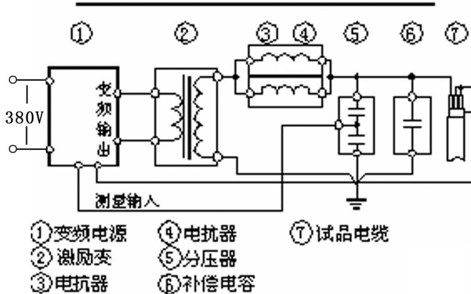
电缆耐压试验接线图
