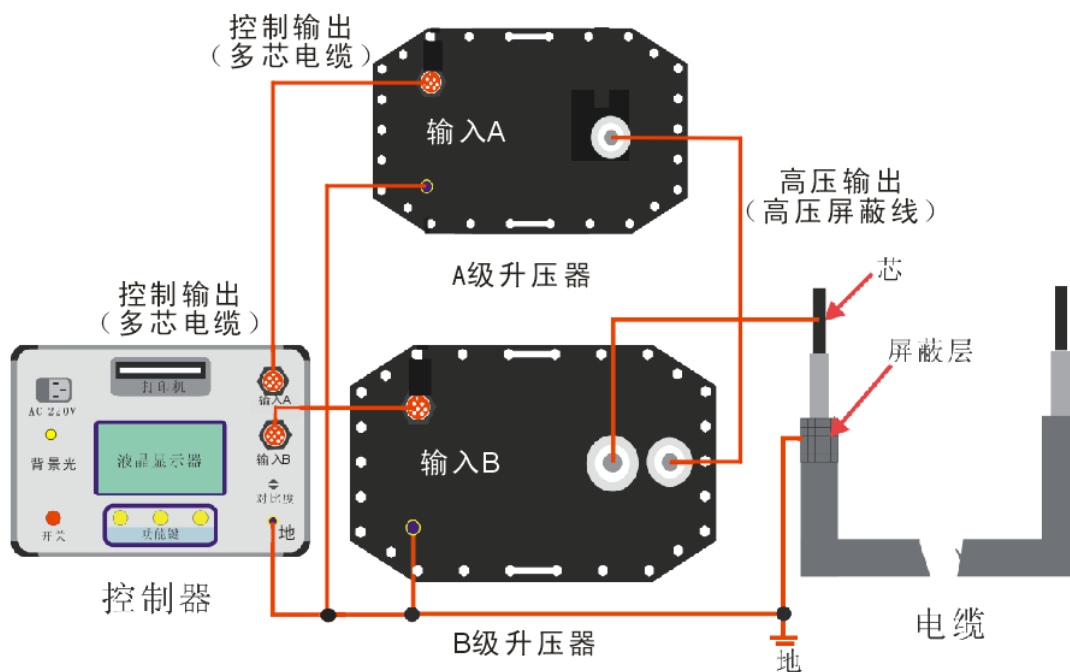
串联连接图
