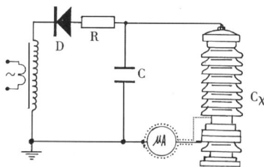
图 b 排除试品 C_x 表面影响接线图
