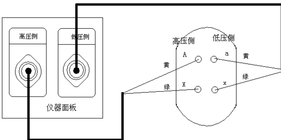
图十九、单相变压器的测试接线
