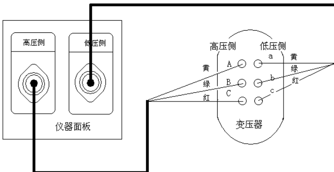
图十八、三相变压器的测试接线
