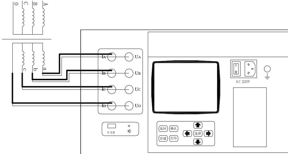
低压侧三相、单相、单线测试接线图
