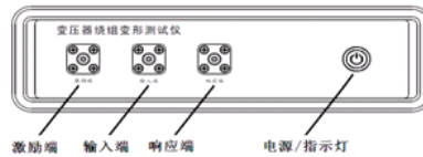
图1a变压器绕组变形测试仪面板图(前面板)
