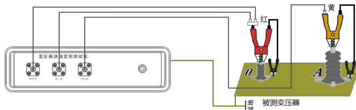
图2 接线示意图
