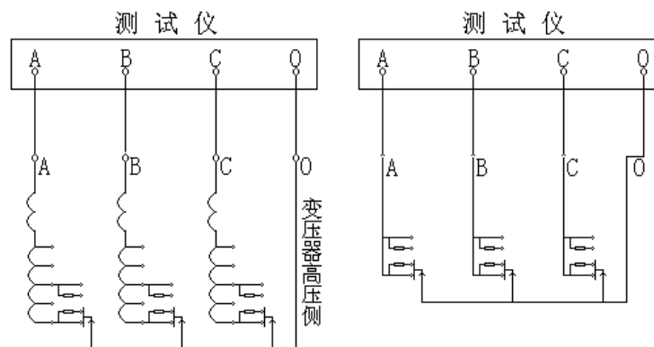
带线圈测量接线图
