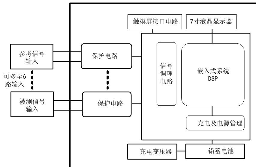
图 1 ED8030 型氧化锌避雷器在线监测及分析系统原理图
