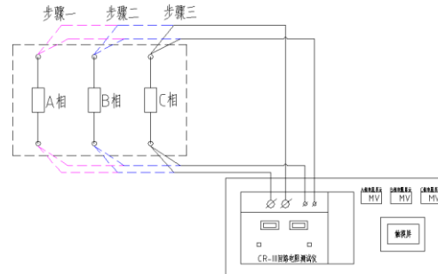
图一、系统原理图
