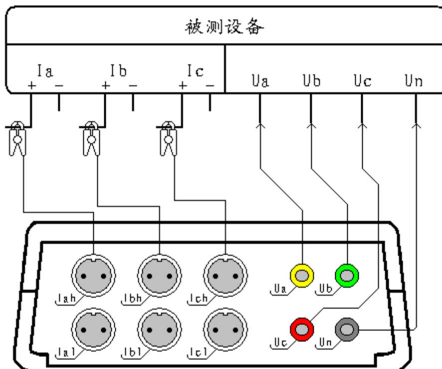
图三十二、频谱分析接线图
