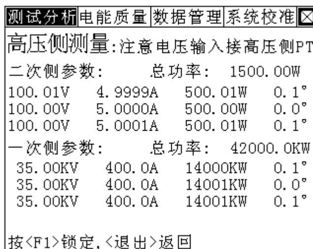
图十一、高压参量
