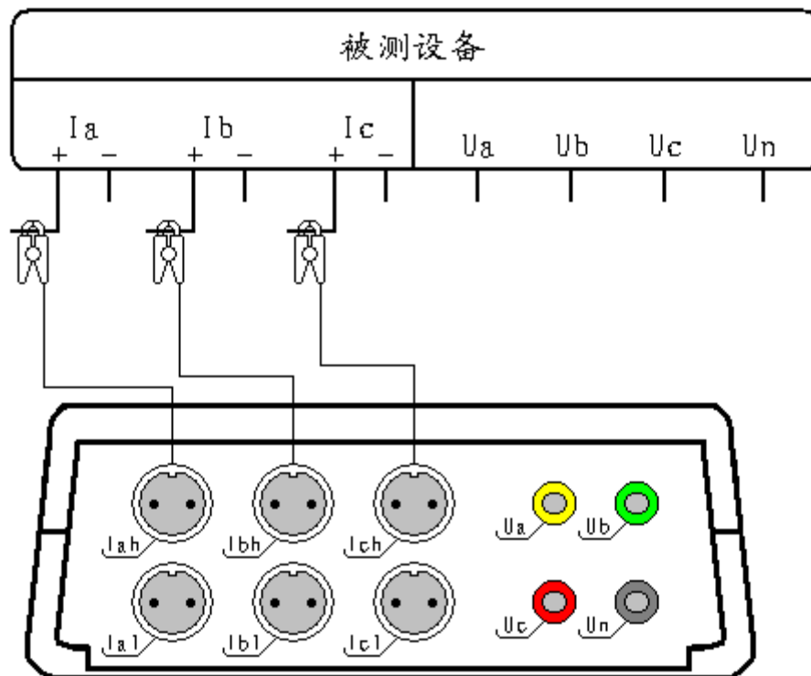
图三十四、电流谐波测试接线图
