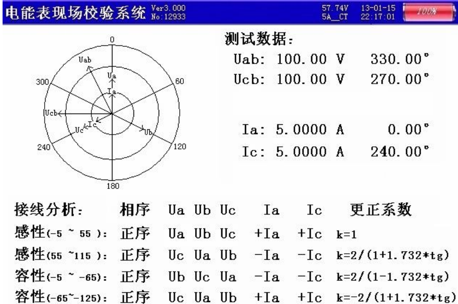
图十、矢量分析屏—三相三线
