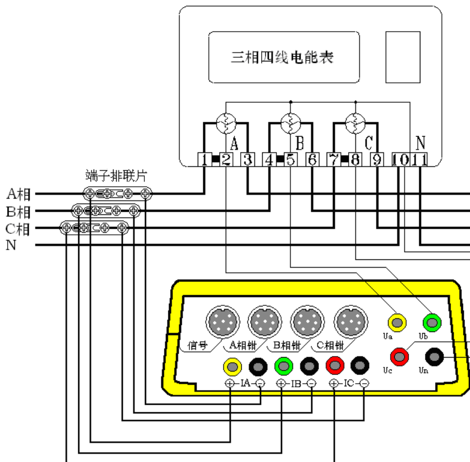
三相四线低压表计经内部CT接入接线
