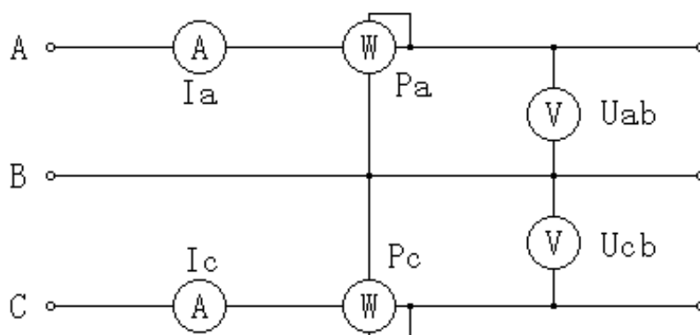
图二十、三相三线制测量原理图
