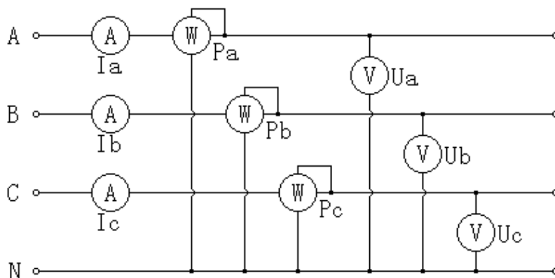
图二十一、三相四线制测量原理图
