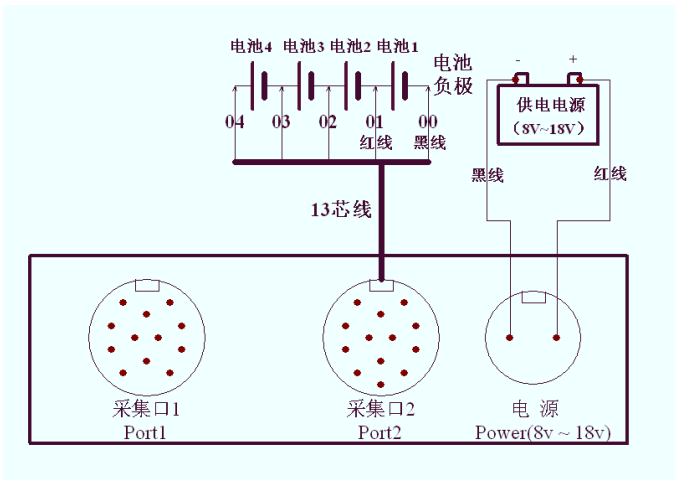
图 2.4.4-2 4 节 12V 电池与 1 个单体模块连接图
