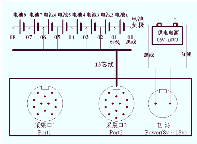
图 2.4.4-1 8 节 6V 电池与 1 个单体模块连接图
