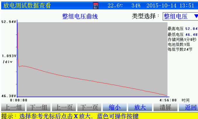
图 3.7.4 整组电压曲线界面
