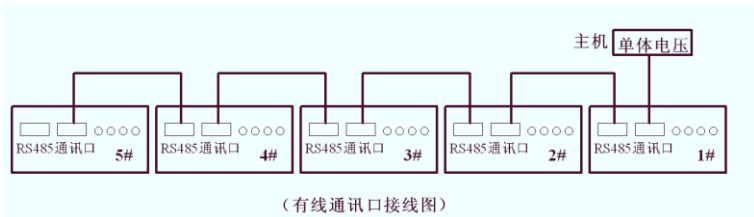
图 2.4.4-4 有线通讯口接线图
