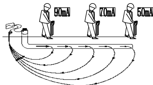
被测管线绝缘不良时探测示意图
