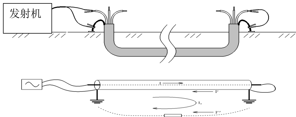
图 4.3 相线 - 护层接法
