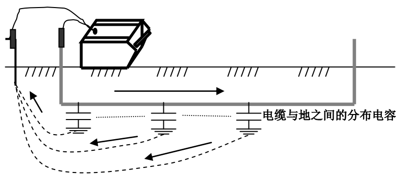
直连法容性回路（终端未接地）— 示意图
