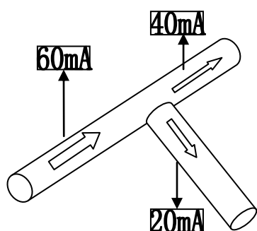
地下管线有三通时的电流值探测示意图
