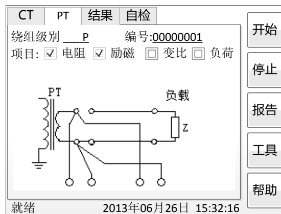
图 2.5 PT 参数设置界面
