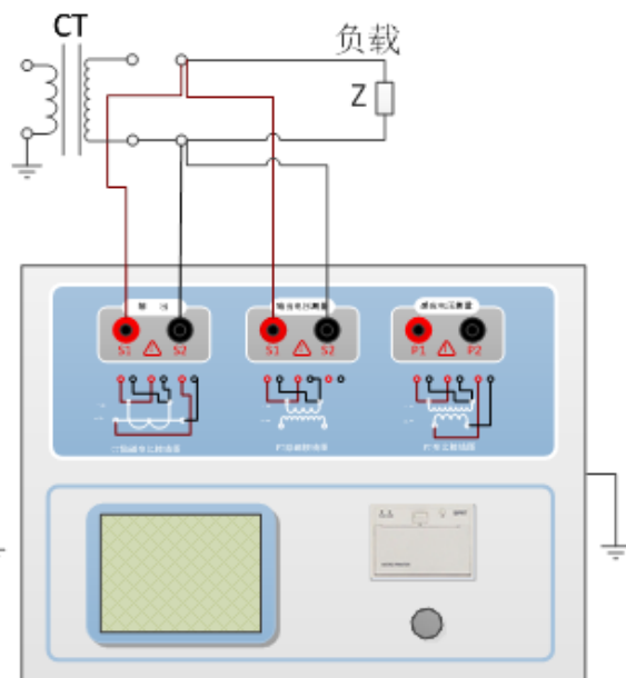
图2.2 CT二次负荷试验接线方式
