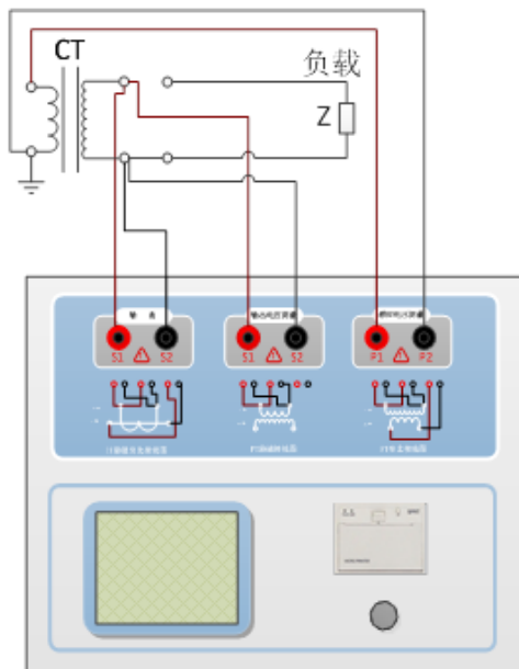
图2.1 CT直阻、励磁、变比试验接线方式
