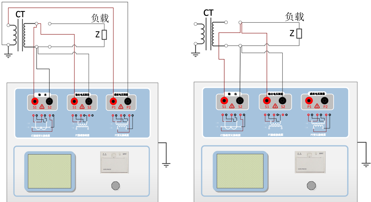
图 2.1 CT 直阻、励磁、变比试验接线方式 图 2.2 CT 二次负荷试验接线方式
