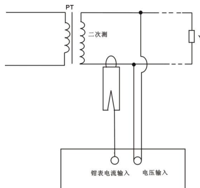
单相 PT 负荷测试接线图
