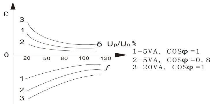
电压互感器电压与负荷特性
