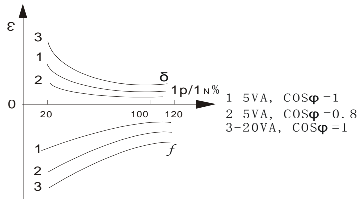
电流互感器的负荷特性曲线
