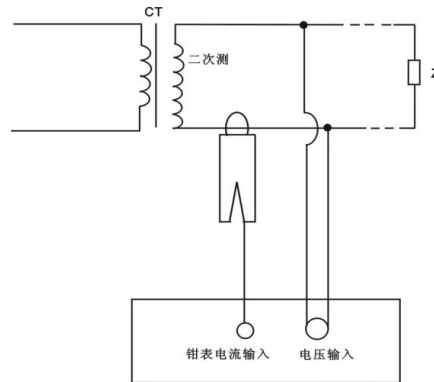
单相 CT 负荷测试接线图
