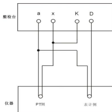
PT 二次压降检定接线图
