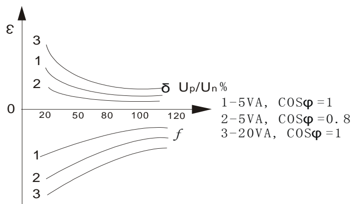
电压互感器电压与负荷特性
