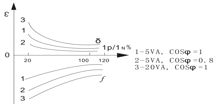
电流互感器的负荷特性曲线
