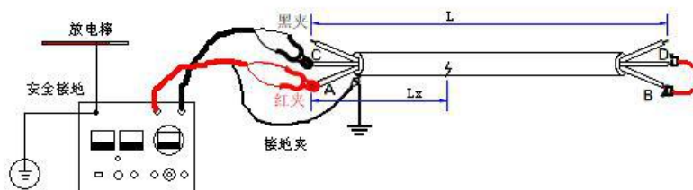
图 5 电桥接线示意图
