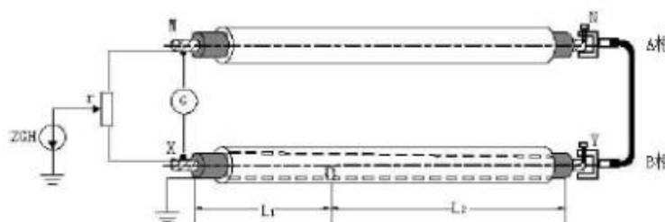
图 6 单芯电缆接线示意图
