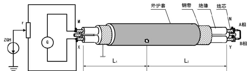
图 3 电桥接线图
