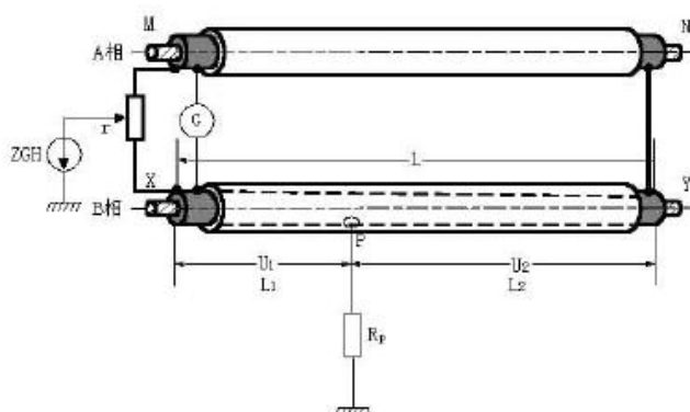
图 7 护层电缆故障接线示意图
