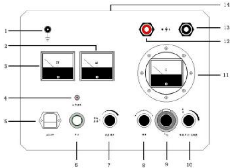
图 1 EDDQ—3 面板示意图
