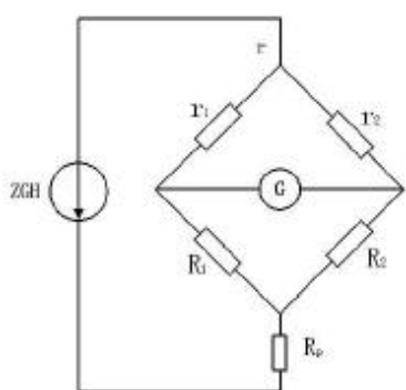
图4 电桥法原理图
