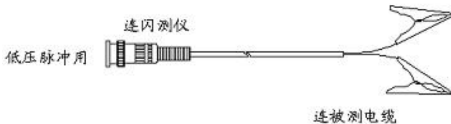
连接电缆示意图
