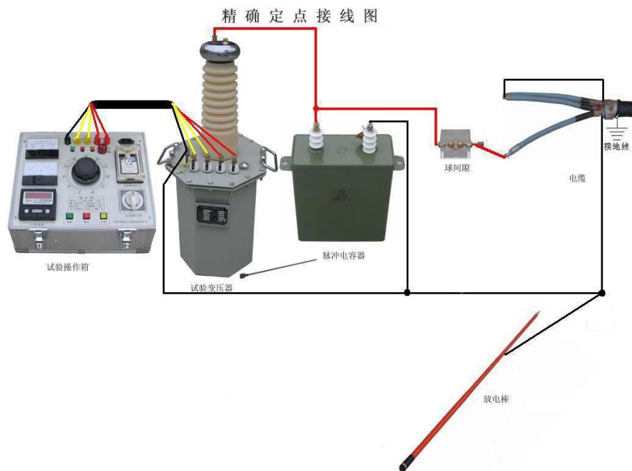
配试验变压器精确定点接线图
