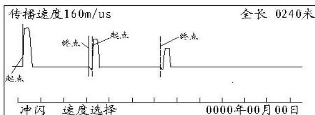
冲闪法电流取样测试波形
