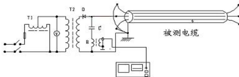
直闪法电流取样接线图
