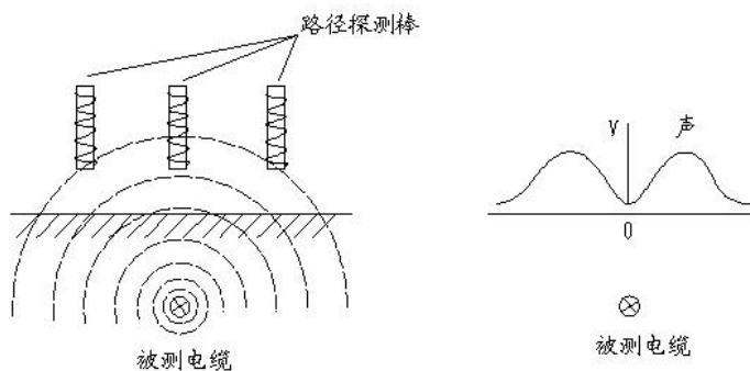
电缆路径探测原理图
