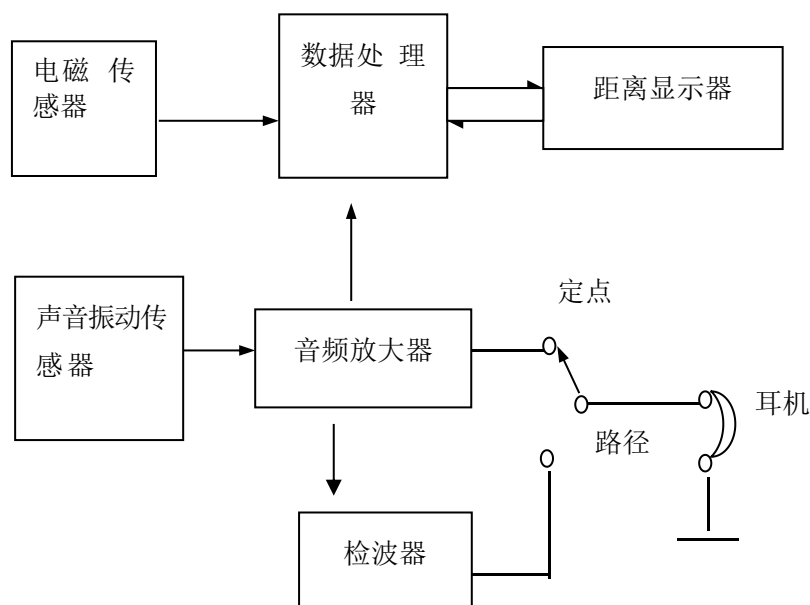
图 2 原理框图
