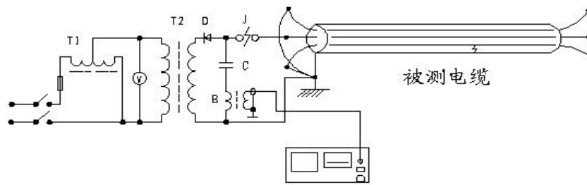
冲闪法电流取样接线图
