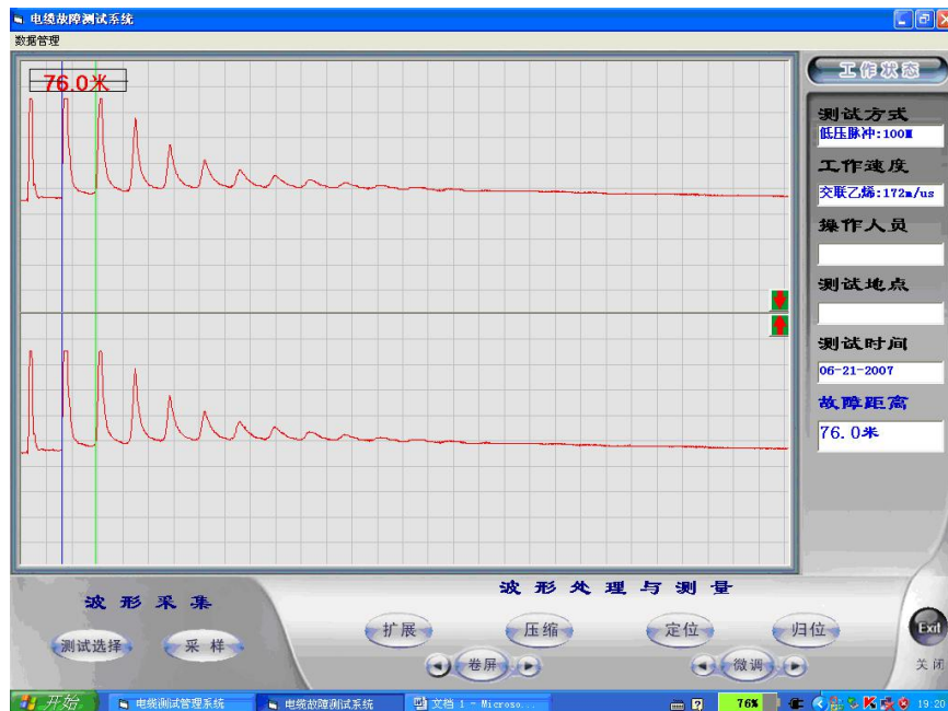
低压脉冲测全长波形(终端开路)
