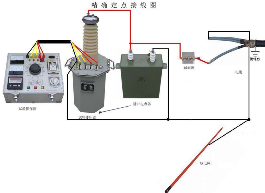
配试验变压器精确定点接线图
