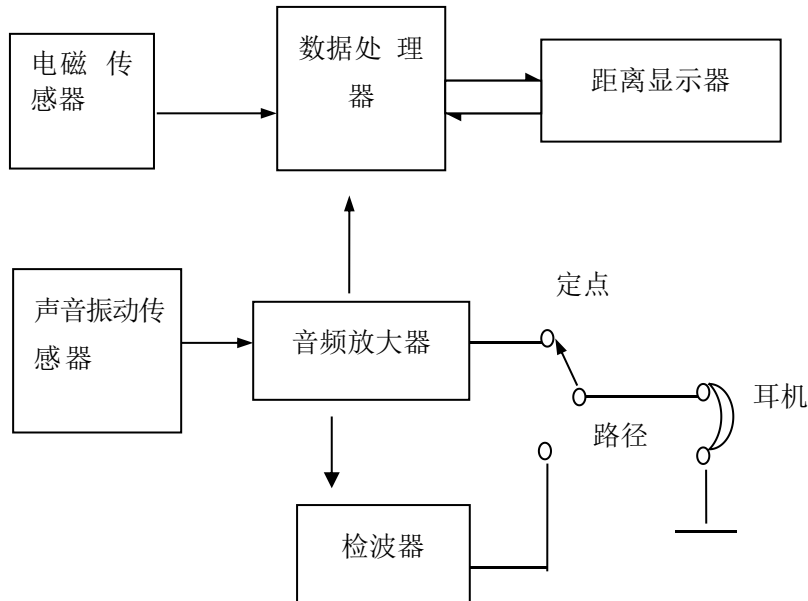
图 2 原理框图
