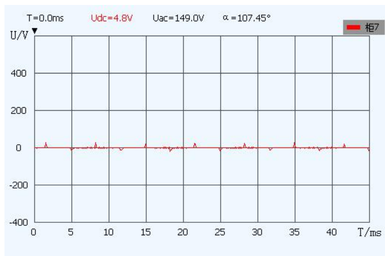
图 14 A+B+C+脉冲断线
