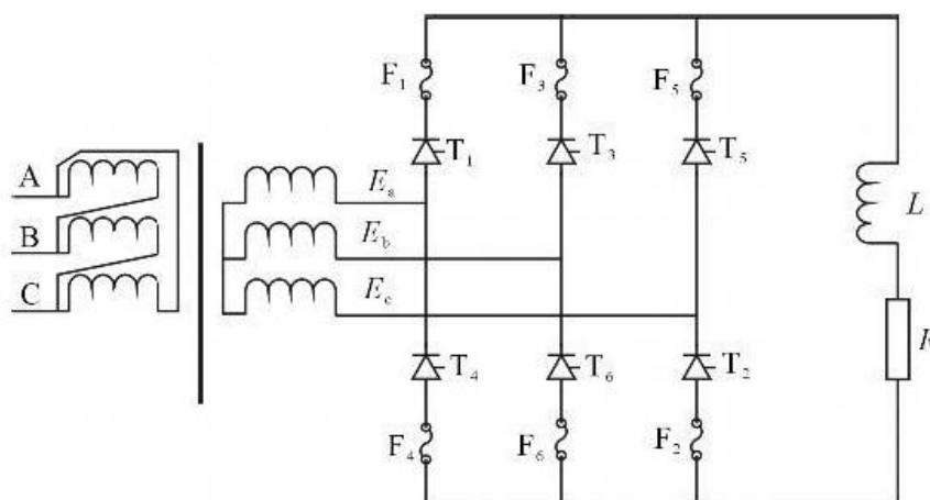
图 7 励磁系统功率单元电路图
