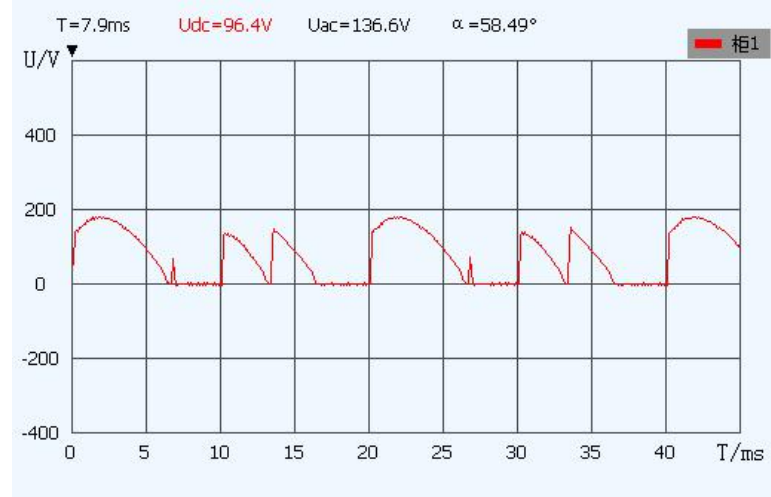
图 15 A+B+脉冲接反
