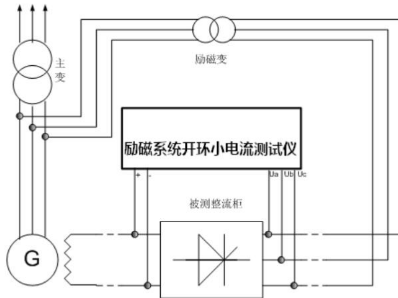
图 1 EDLC-II 型励磁系统开环小电流测试仪测试原理图
