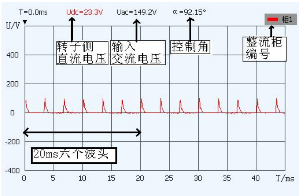
图 4 励磁系统开环小电流试验典型波形图
