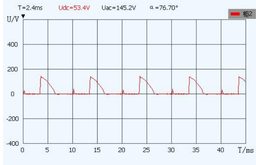
图 9 A+A-脉冲断线
