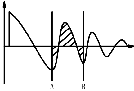
图 1-4-1 波形面积的差比较 (实线是标准波形虚线是实测波)
