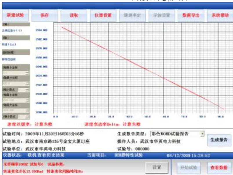
图 10 静特性试验结果
